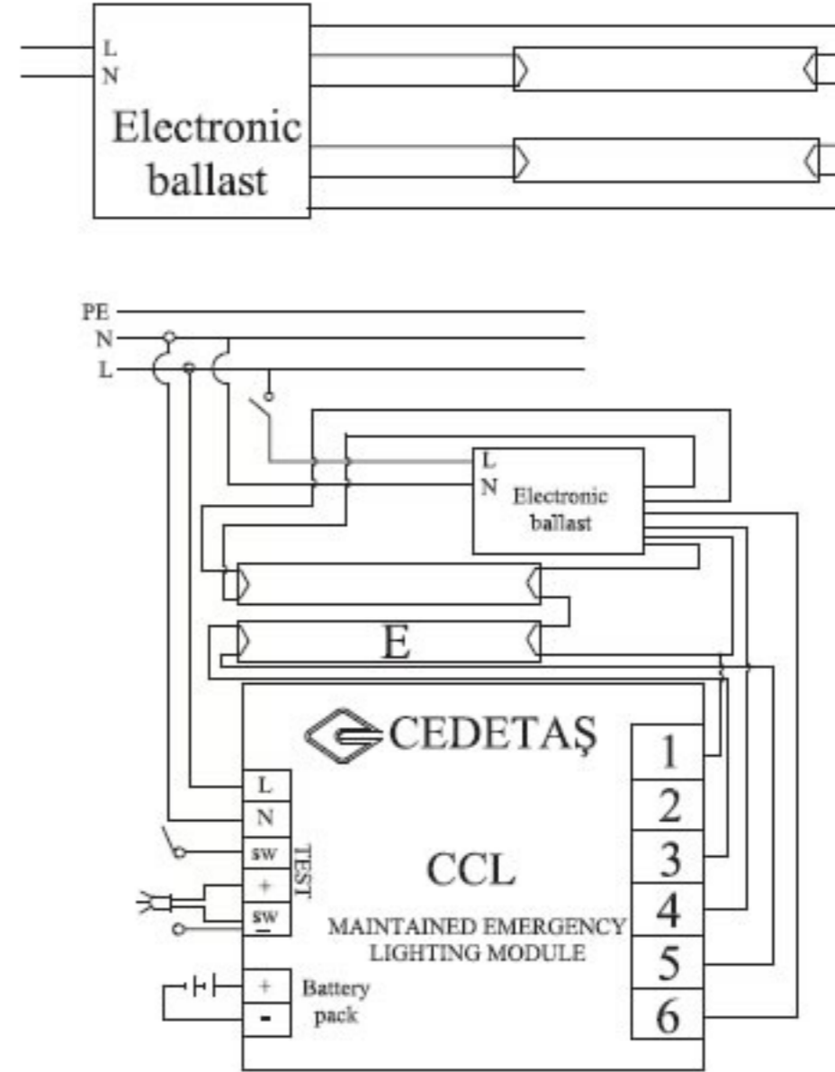
Elektronik Balast Sürekli Mod (1Ballast 2 Lamba)
