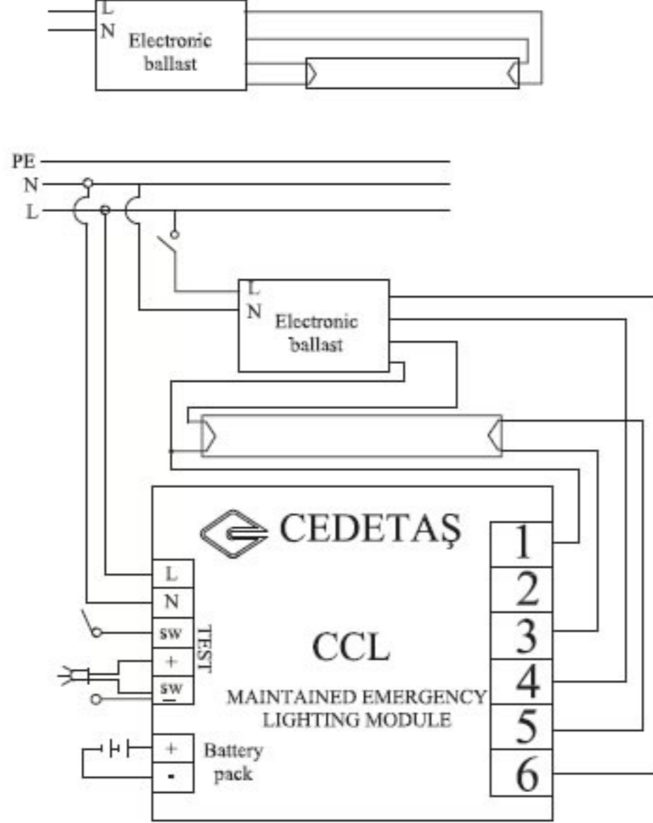
Elektronik Balast Sürekli Mod (1Ballast 1 Lamba)
